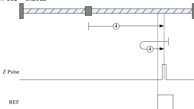
图 5-16 原点回归方式 4
