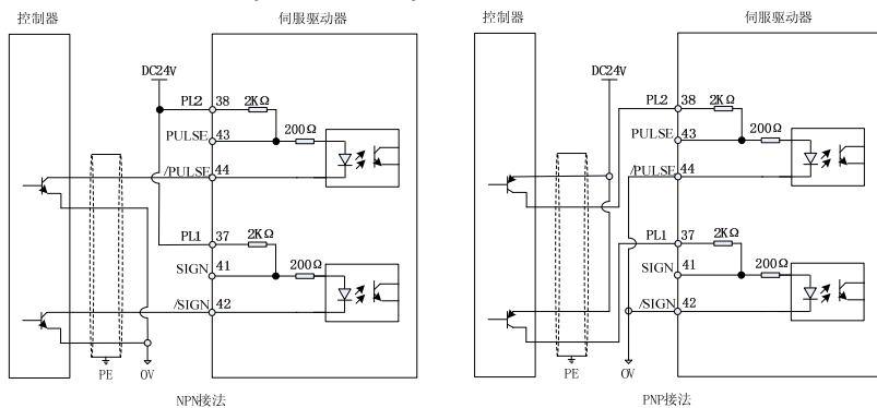
图3-8 集电极开路脉冲指令输入接线图（外部24V）
