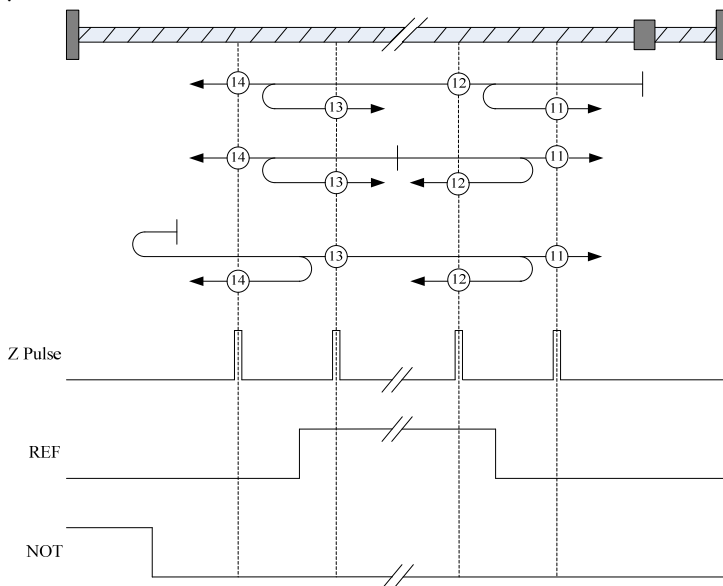
图 5-20 原点回归方式 11/12/13/14
