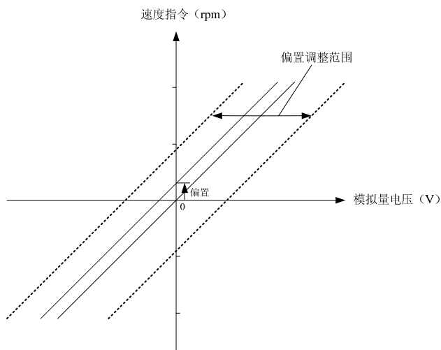
图 5-7 模拟量指令偏置
