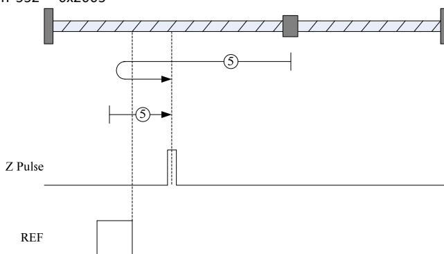
图 5-17 原点回归方式 5
