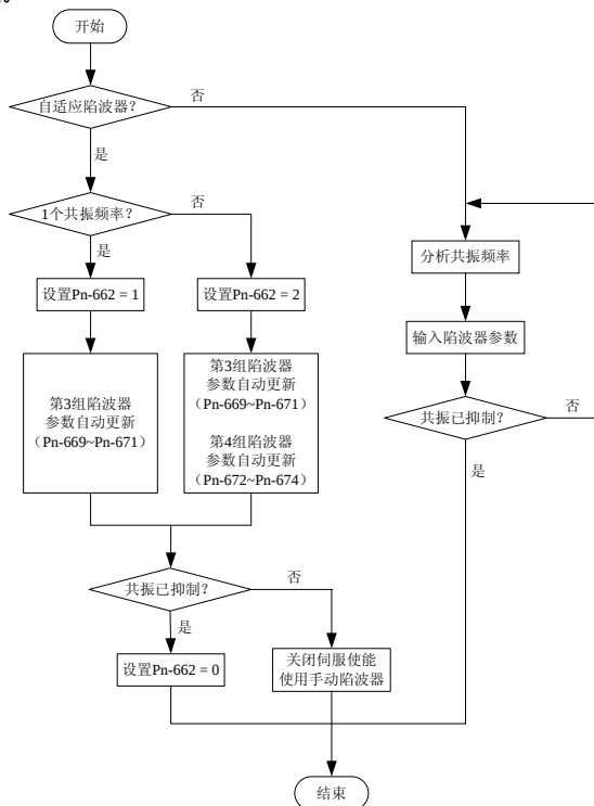
图 6-5 陷波器功能
