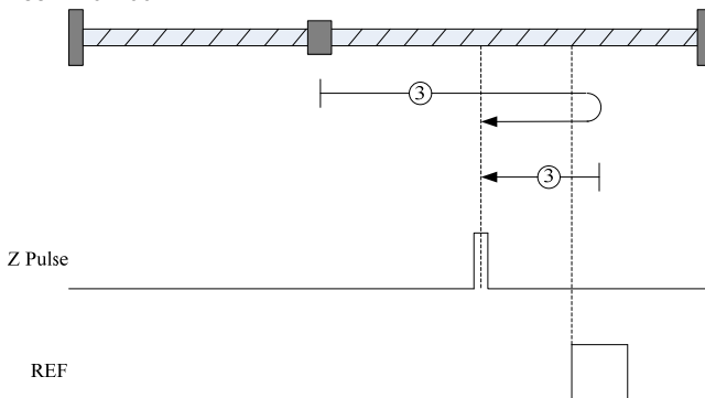
图 5-15 原点回归方式 3
