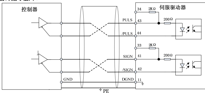
图3-6 差分脉冲指令输入接线图
