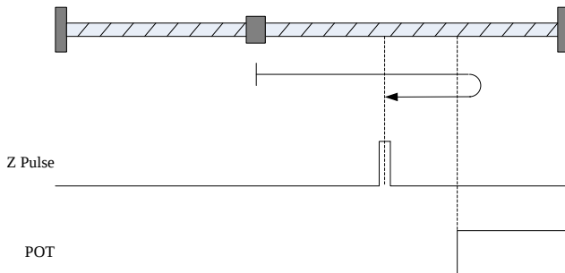
图 5-14 原点回归方式 2
