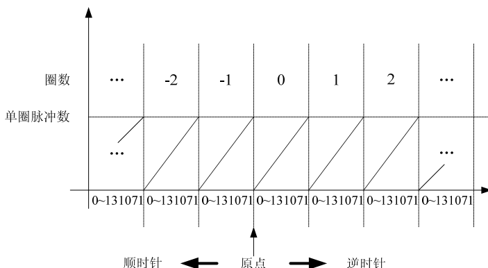
图 5-23 脉冲数值计数方式
