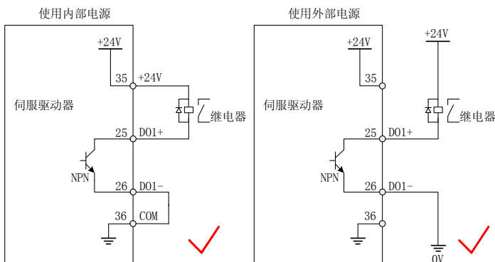
图3-13 数字量输出端子连接继电器时正确接线
