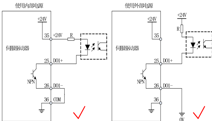
图3-15 数字量输出端子连接光耦时正确接线
