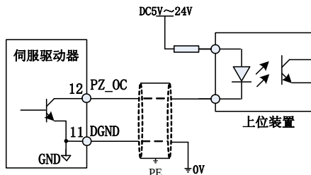
图3-18 编码器（集电极开路输出）与上位装置连线
