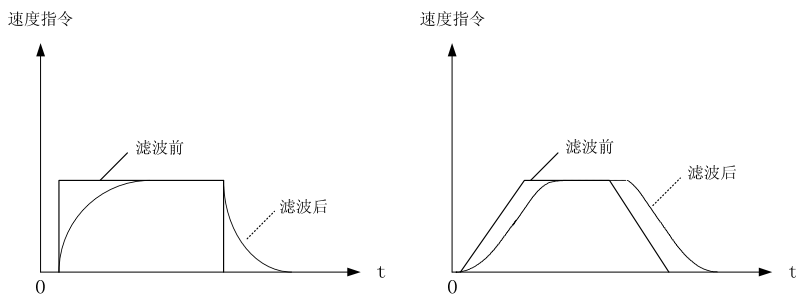
图 5-6 模拟量指令滤波
