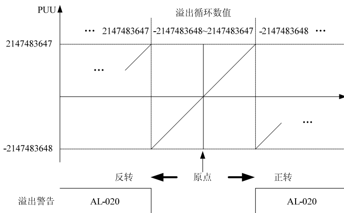
图 5-24 PUU 数值计数方式
