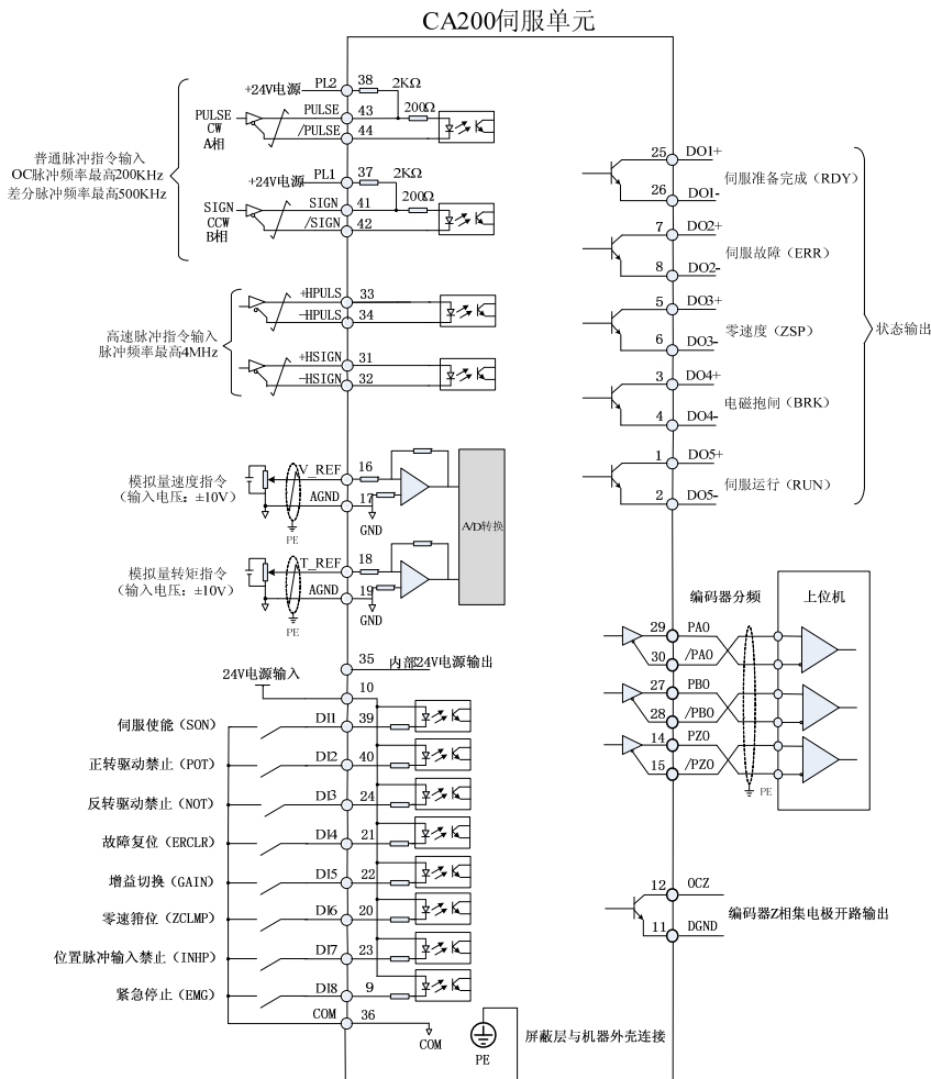
图3-5 位置/速度/转矩控制接线图
