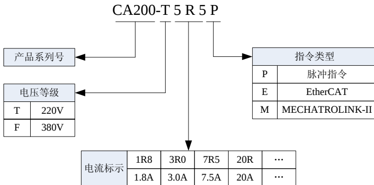
图 1-1 伺服驱动器型号说明
