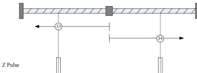
图 5-22 原点回归方式 33/34
