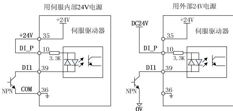
图3-11 上位装置为集电极开路（NPN）输出时的数字输入接线图
