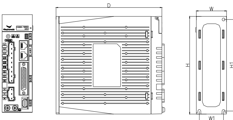
图2-1 伺服驱动器安装方法
