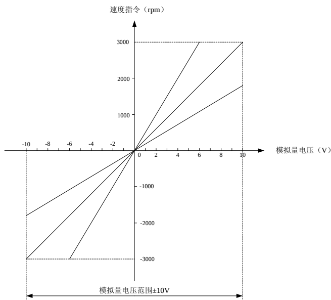
图 5-6 模拟量指令比例
