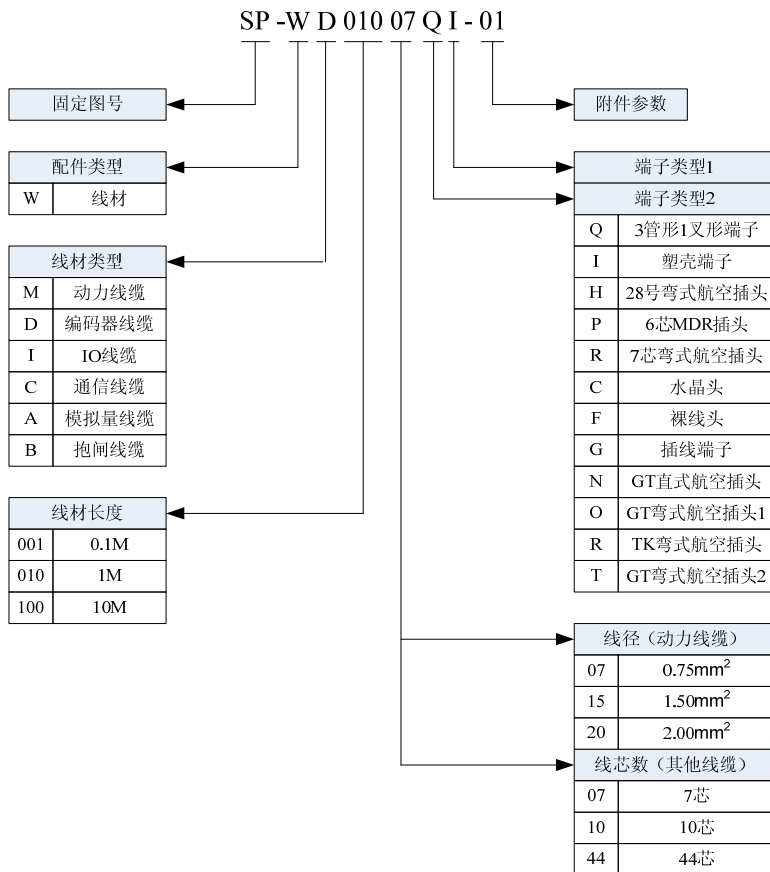
图 10-1 伺服线缆命名规则
