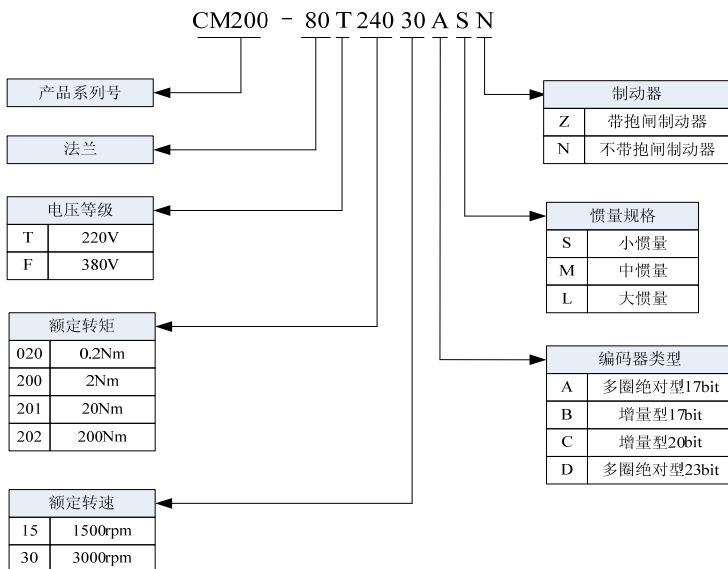
图 1-2 伺服电机型号说明
