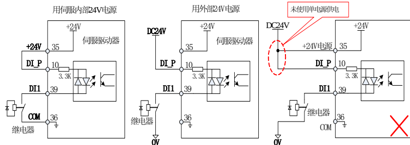
图3-10 上位装置为继电器输出时的数字输入接线图
