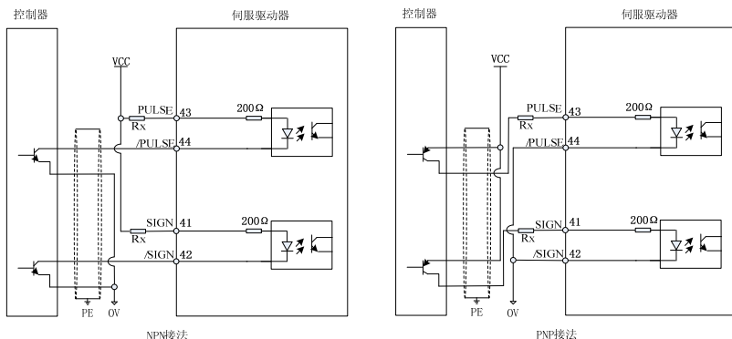
图3-9 集电极开路脉冲指令输入接线图（外部VCC）
