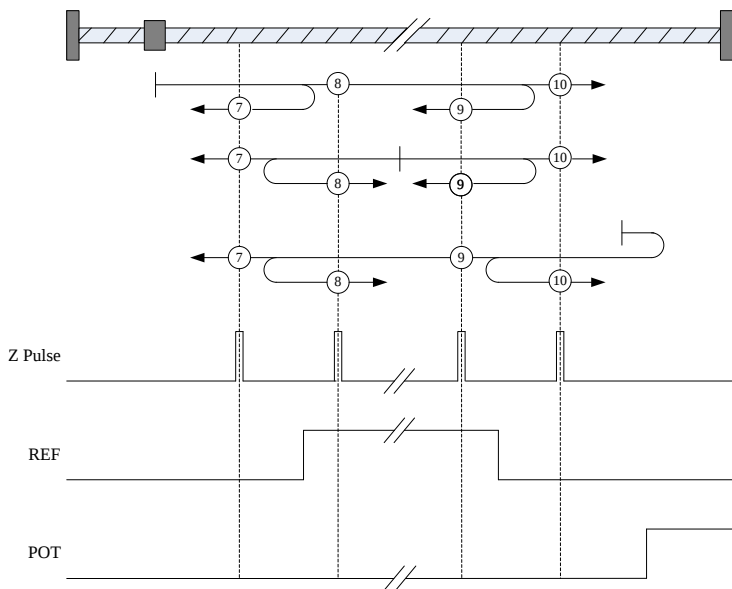
图 5-19 原点回归方式 7/8/9/10
