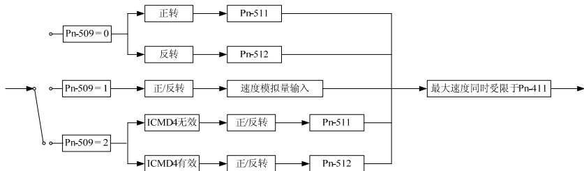
图 5-12 转矩模式下速度限制
