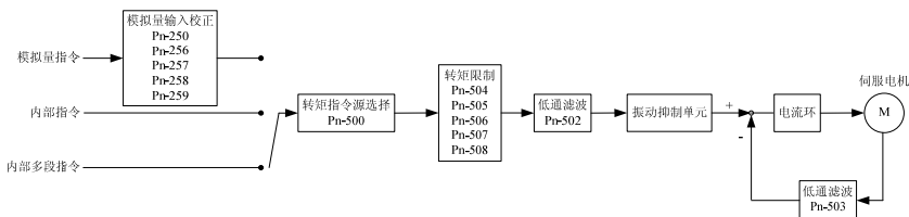
图 5-10 转矩控制
