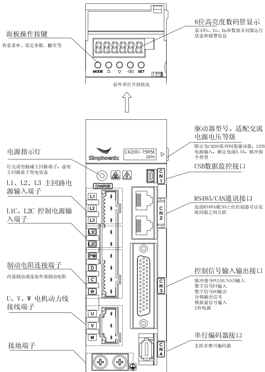
图 1-3 驱动器各部分名称
