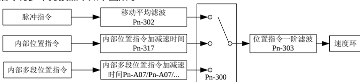
图 6-4 滤波器
