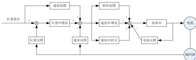
图 6-3 伺服控制环路
