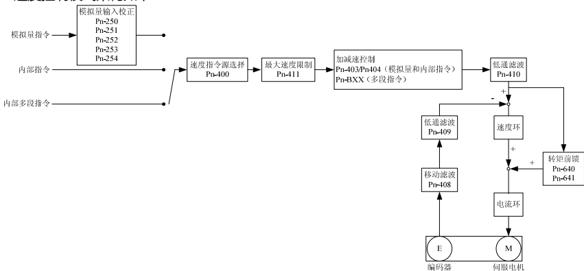
图 5-5 速度控制
