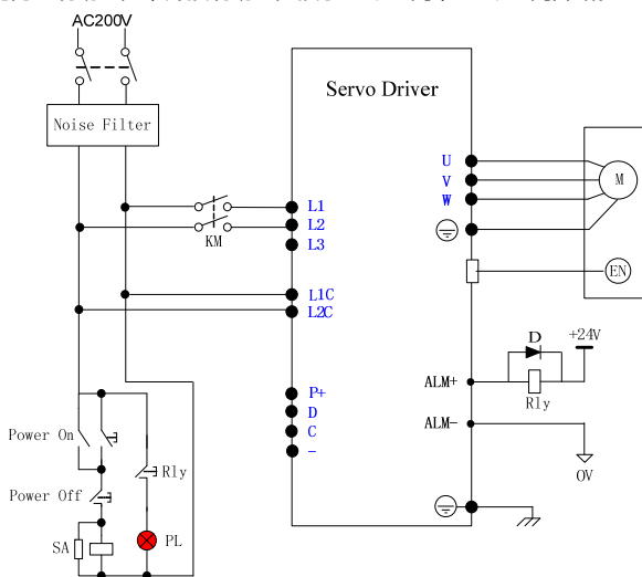
图 3-2 单相 220V 主回路接线示意
