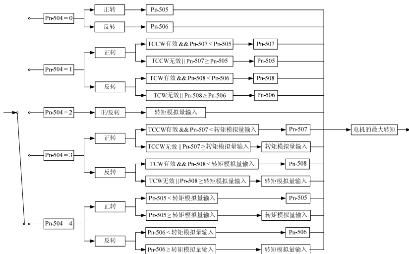
图 5-11 转矩限制
