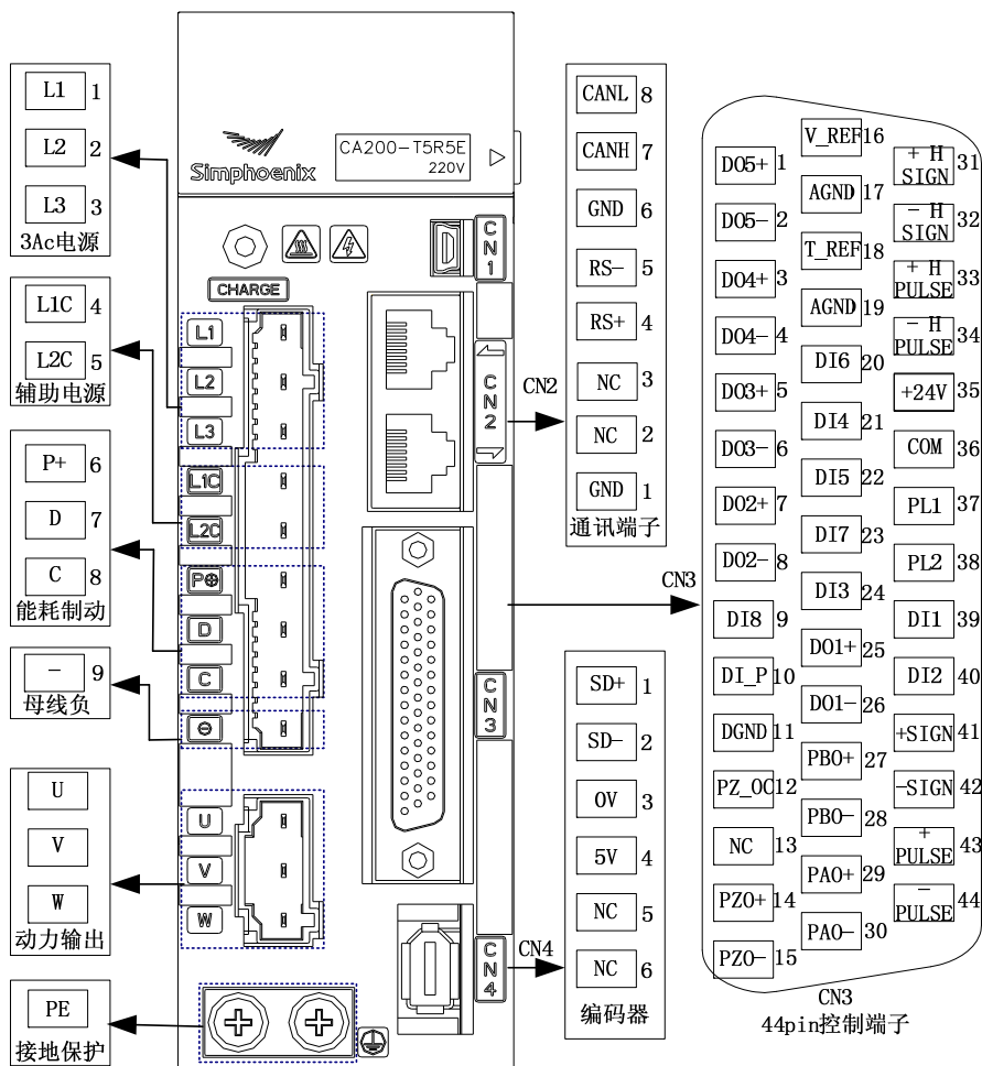
图 1-4 伺服驱动器端子引脚分布图
