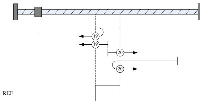
图 5-21 原点回归方式 19/20
