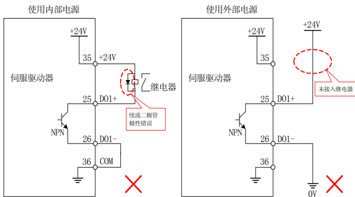
图3-14 数字量输出端子连接继电器时错误接线
