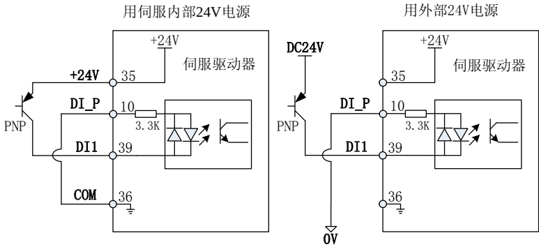
图3-12 上位装置为集电极开路（PNP）输出时的数字输入接线图
