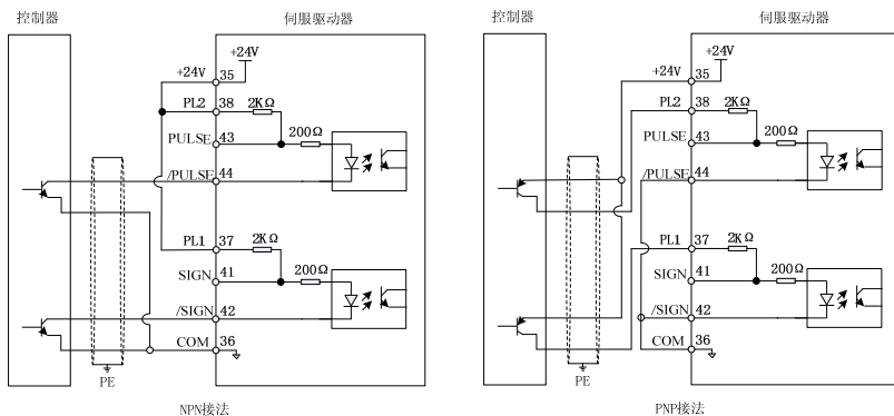
图3-7 集电极开路脉冲指令输入接线图（内部24V）
