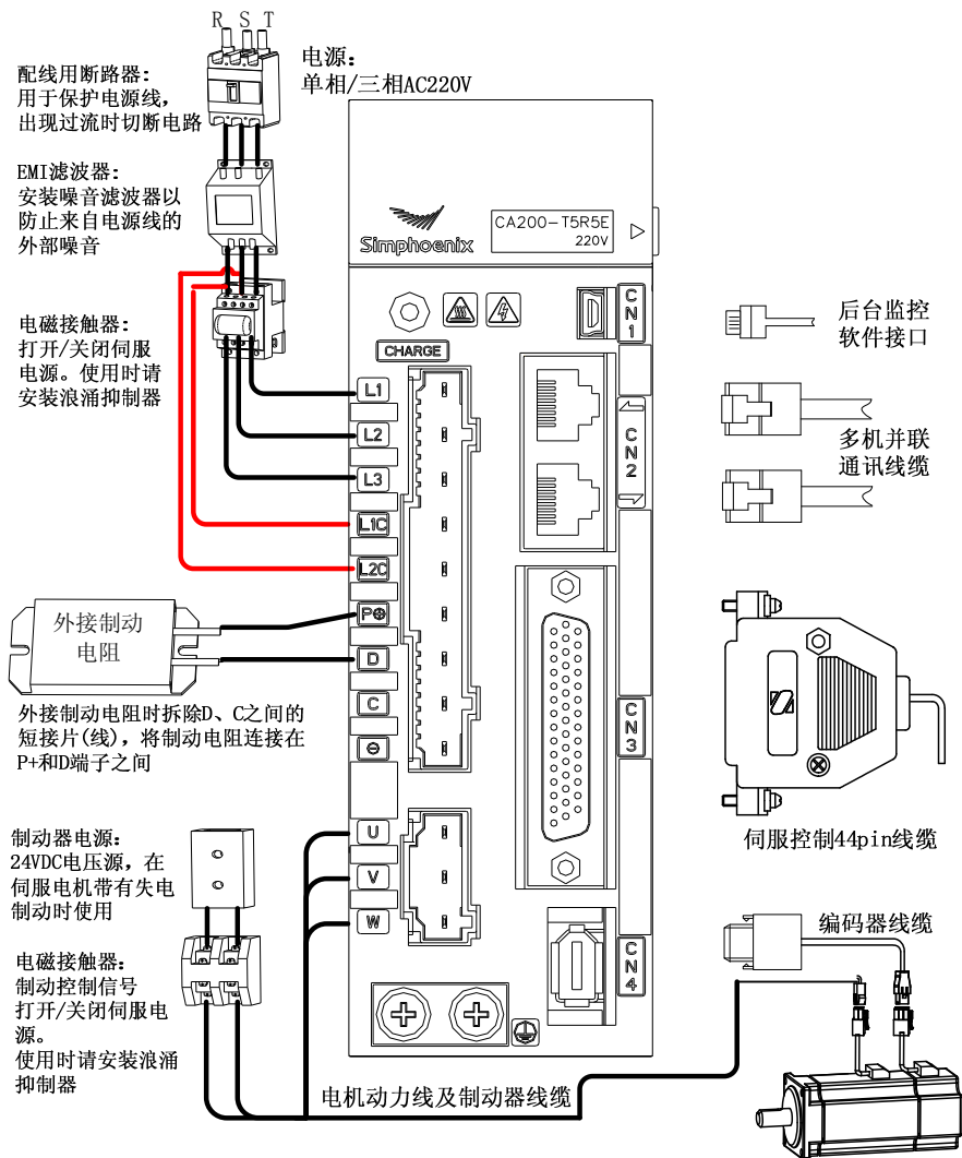
图 3-1 伺服驱动器配线图
