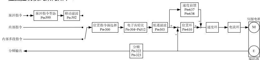
图 5-3 位置控制
