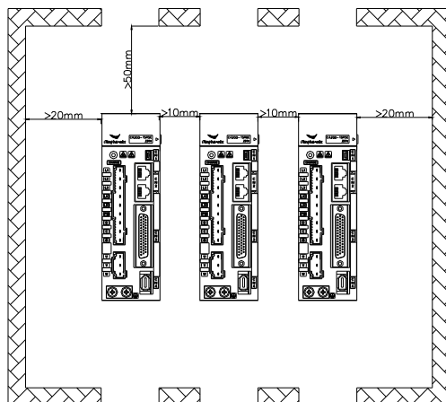
图2-1 伺服驱动器安装方法
