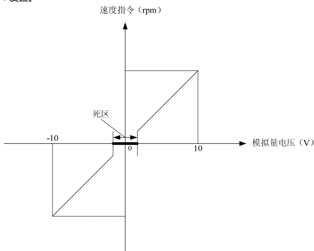
图 5-8 模拟量指令死区
