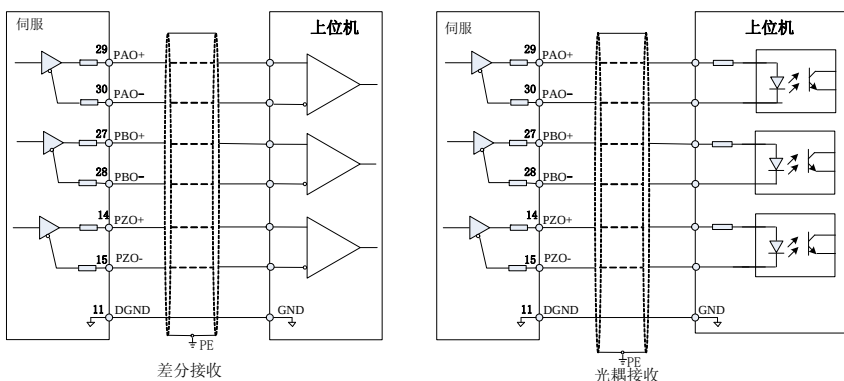
图3-17 编码器分频输出与上位装置连线
