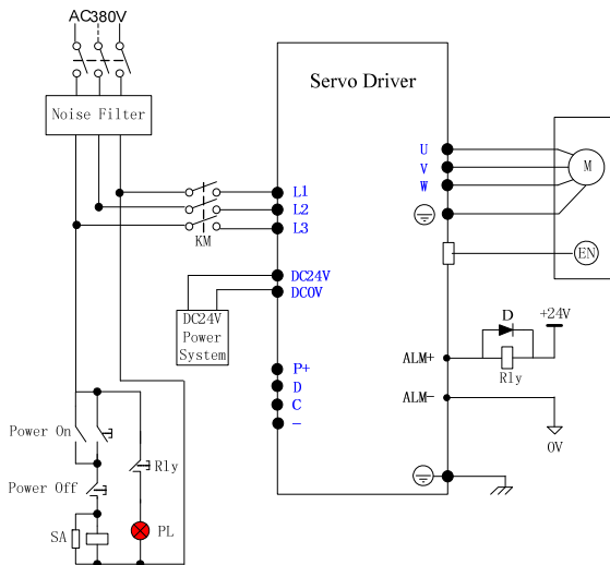
图 3-4 三相 380V 主回路接线示意
