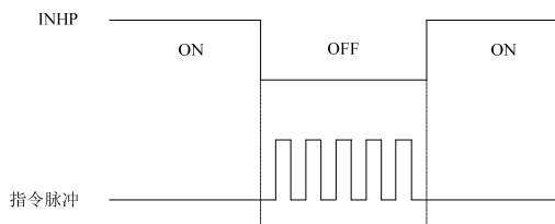
图 5-4 脉冲禁止功能
