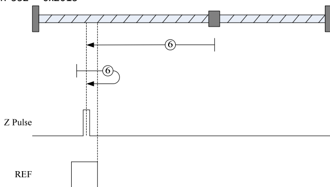
图 5-18 原点回归方式 6
