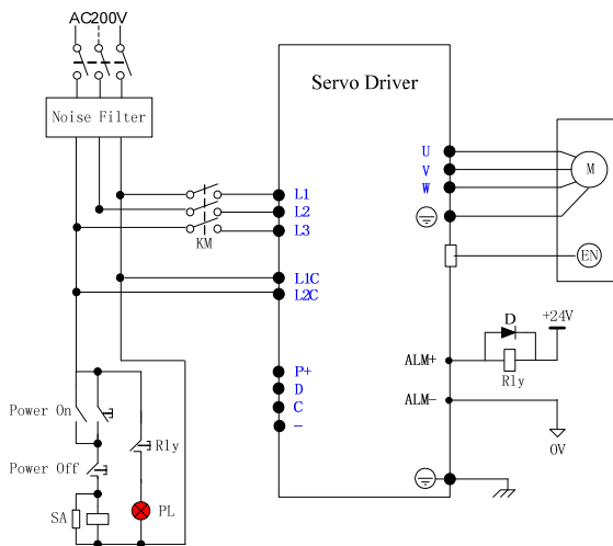
图 3-3 三相 220V 主回路接线示意
